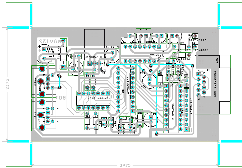
NAVIGATOR-1 plan osazení součástek na plošném spoji
